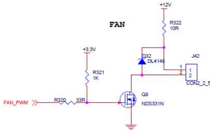
图 3-19-1 开发板原理图中风扇设计
