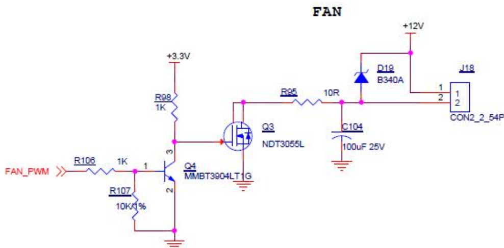
图 3-19-1 开发板原理图中风扇设计
