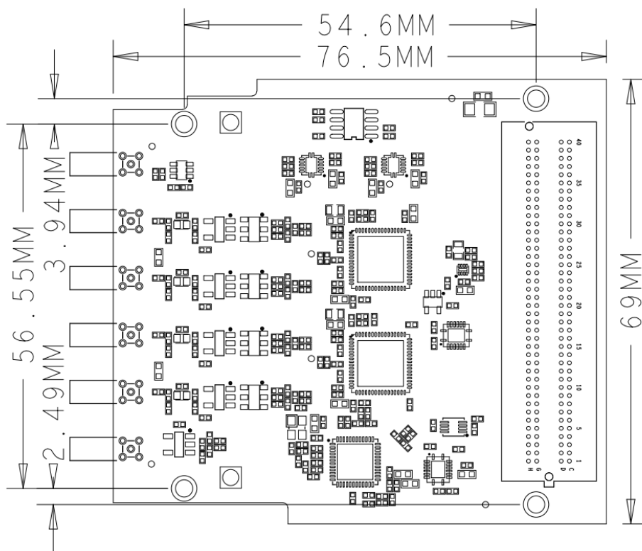
FL2512 高速 AD 模块尺寸结构图
