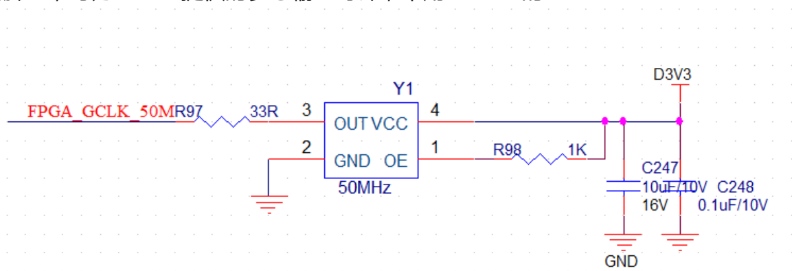
图 2-3-5 50Mhz 有源晶振
