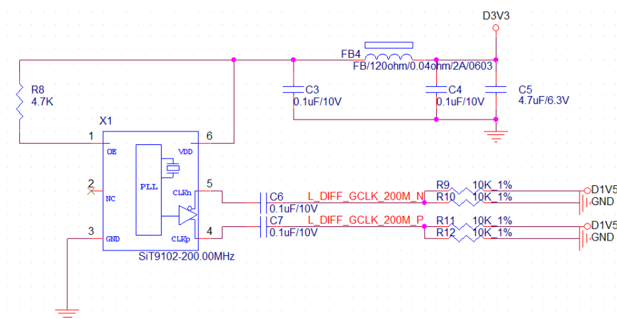
图 2-3-1 200M 有源差分晶振
