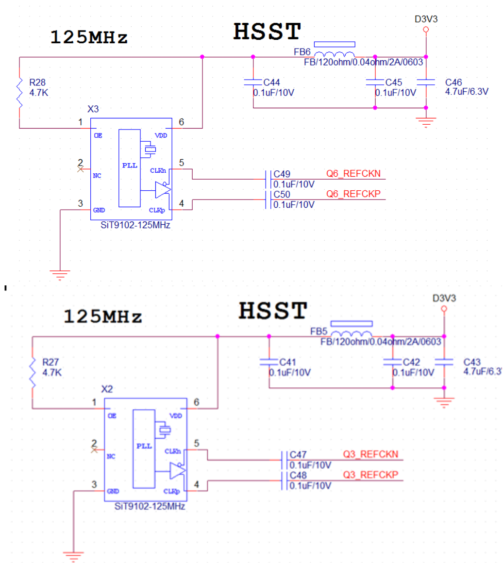
图 2-3-3 125Mhz 有源差分晶振
