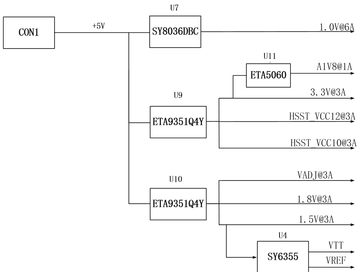
图 1-8-1 原理图中电源接口部分
