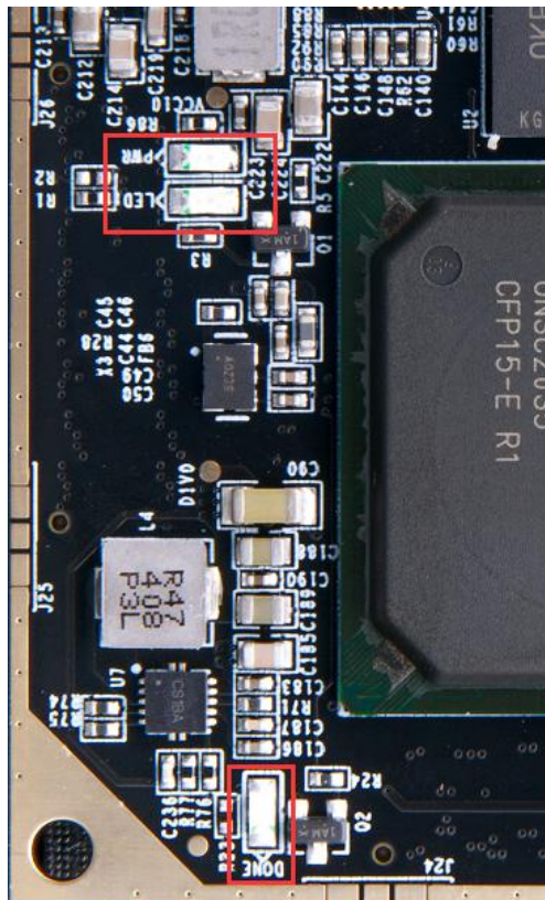
图 1-6-2 核心板的 LED 灯实物图
