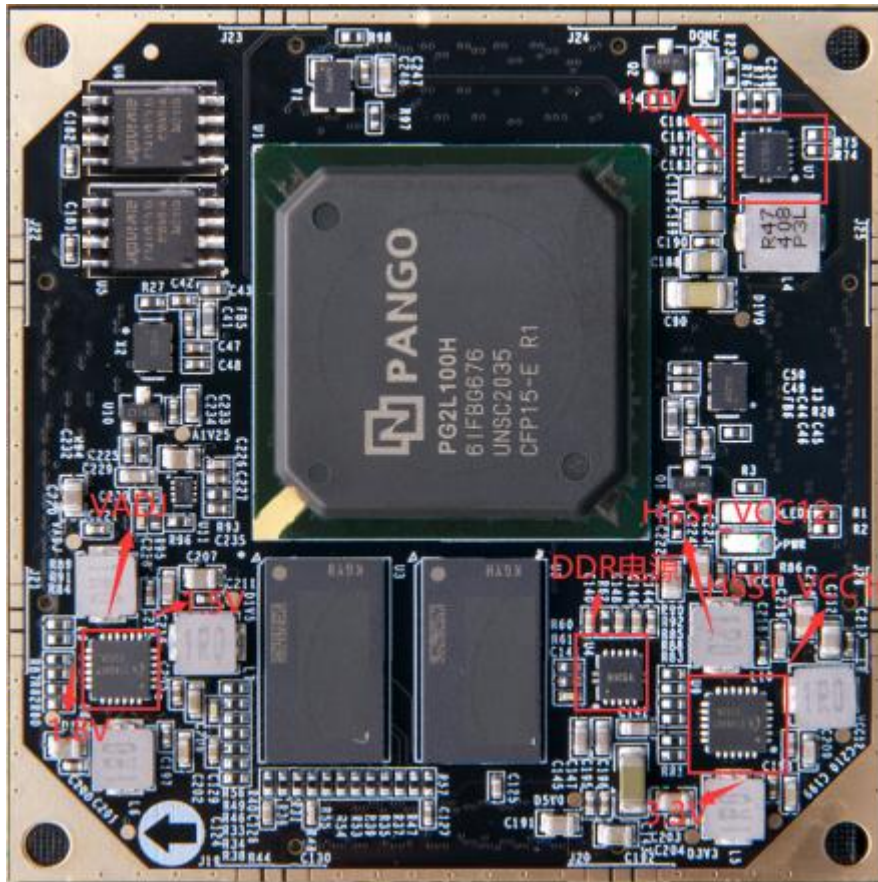
图 1-8-2 核心板电源部分实物图
