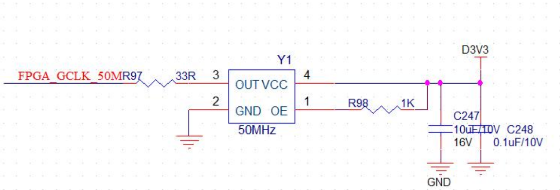
图 1-3-5 50Mhz 有源晶振
