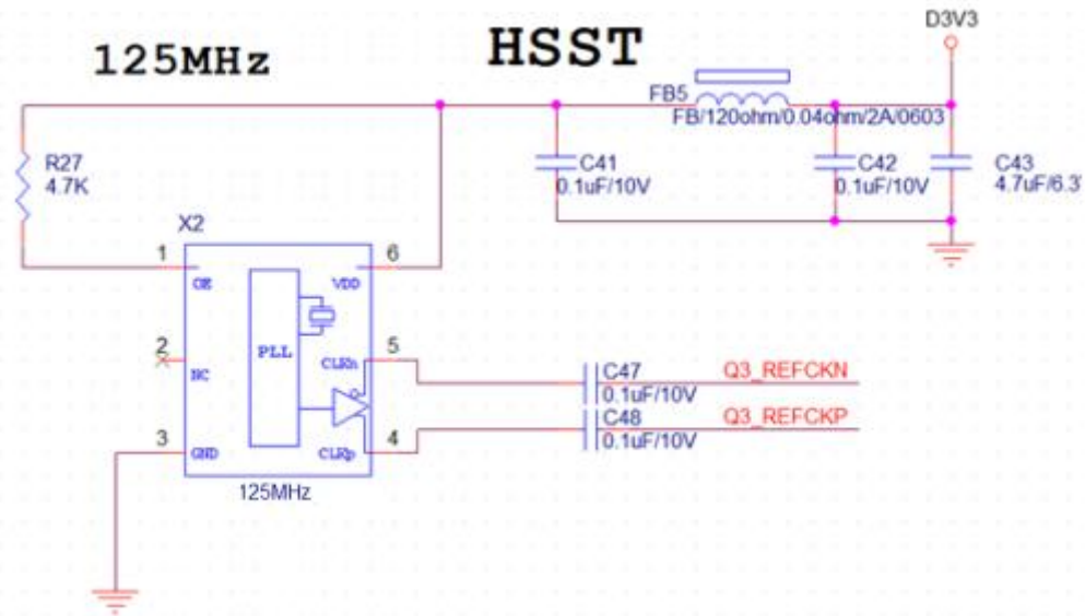
图 1-3-3 125Mhz 有源差分晶振
