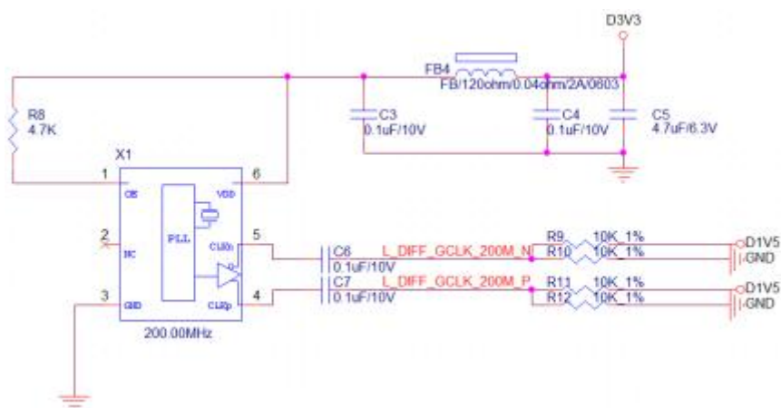
图 1-3-1 200M 有源差分晶振
